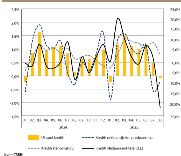
G13: Mjesečna promjena kredita
