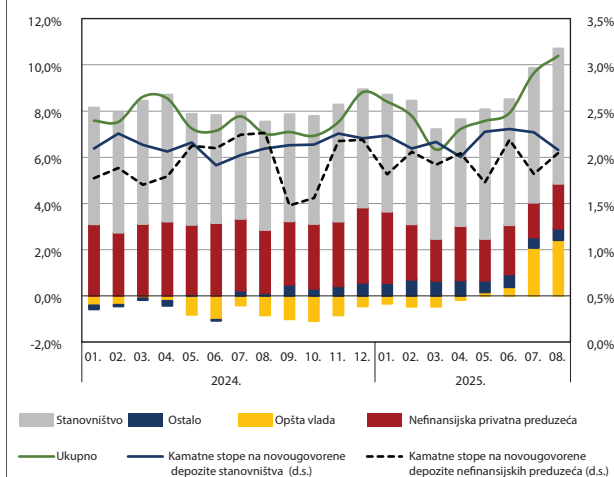
G14: Doprinosi godišnjoj promjeni ukupnih depozita i kamatne stope na novougovorene depozite
