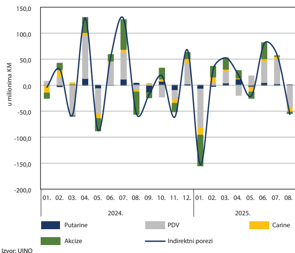
G16: Mjesečne promjene indirektnih poreza
