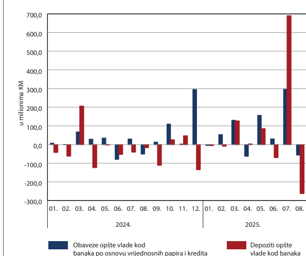
G15: Obaveze i depoziti opšte vlade kod komercijalnih banaka, mjesečne promjene
