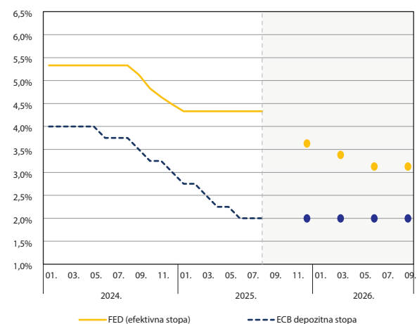
G02: Referentne stope vodećih centralnih banaka
