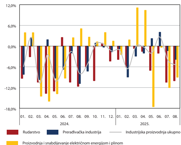
G06: Godišnje promjene obima industrijske proizvodnje po područjima, izvorni indeksi
