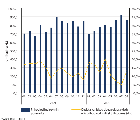
G17: Otplata vanjskog duga sektora opšte vlade
