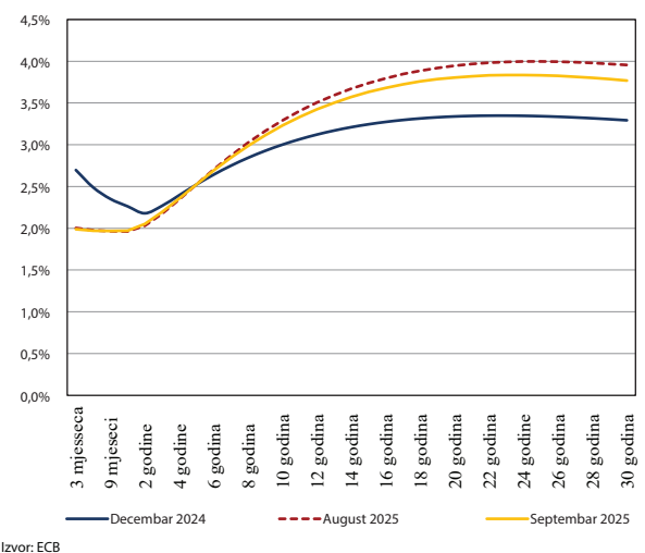
G03: Kriva prinosa u eurozoni
