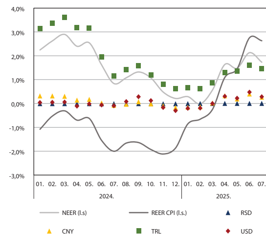
G04: Godišnje promjene u deviznom kursu
